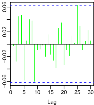
(d) ACF of squared residuals
