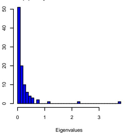
(d) Projection of Factor Model
