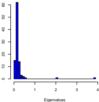
(d) Projection of Factor Model
